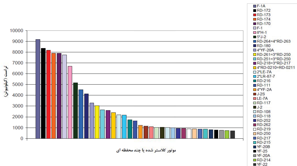
شکل (۱): محدوده نیروی پیشران موتورهای مورد بررسی [۱۵].
