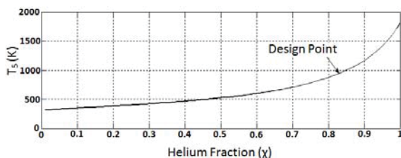
شکل (۹): درصد ترکیب هلیوم (رابطه (۱)) برای برقراری شرط طراحی.
