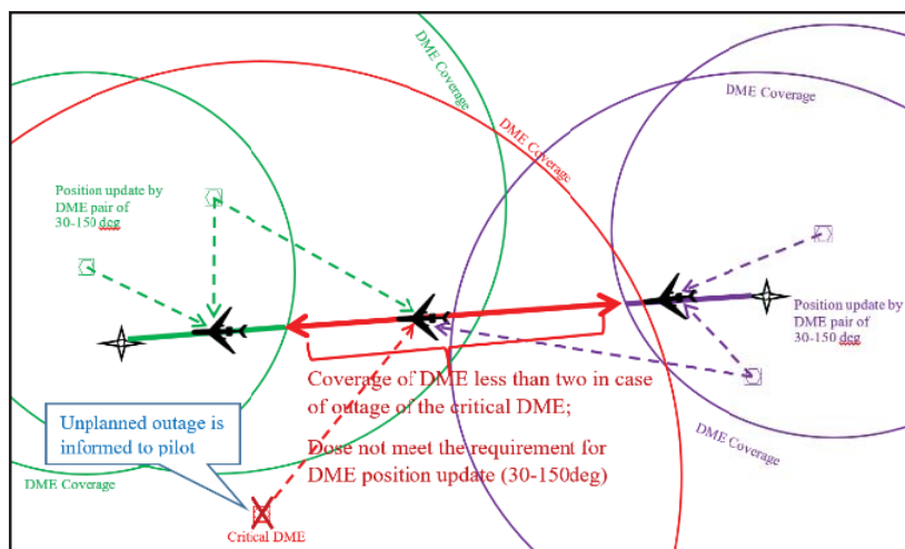
شکل (۱۲): DME بحرانی [۹].
