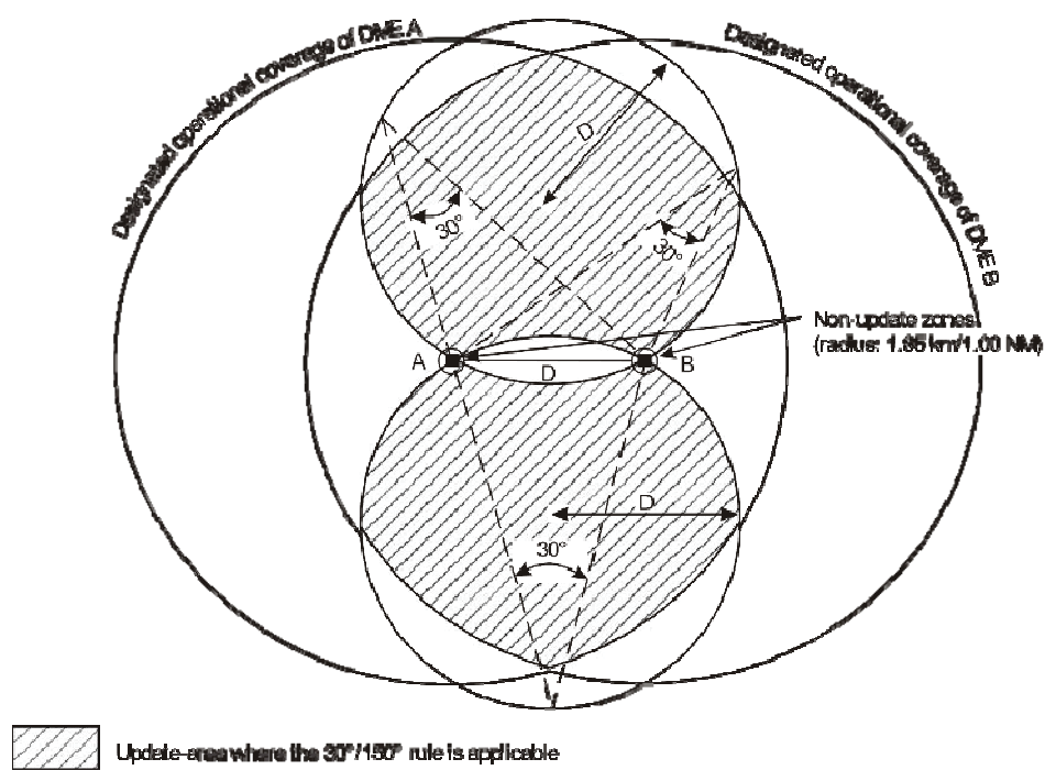
شکل (۹): پوشش DME/DME [۱۱].
