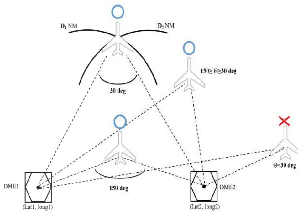
شکل (۸): محدوده مجاز زاویه تقاطع دو ایستگاه DME [۷].
