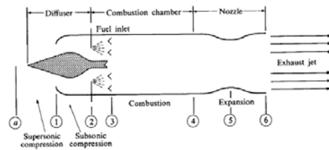
شکل (۱): شماتیک موتور پیشران رمجت [۱۶].
