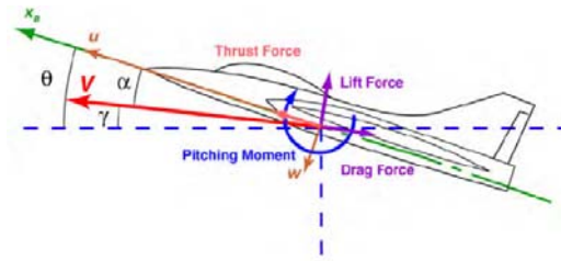
شکل (۲): شمایک وسیله پرنده [۲۶].
