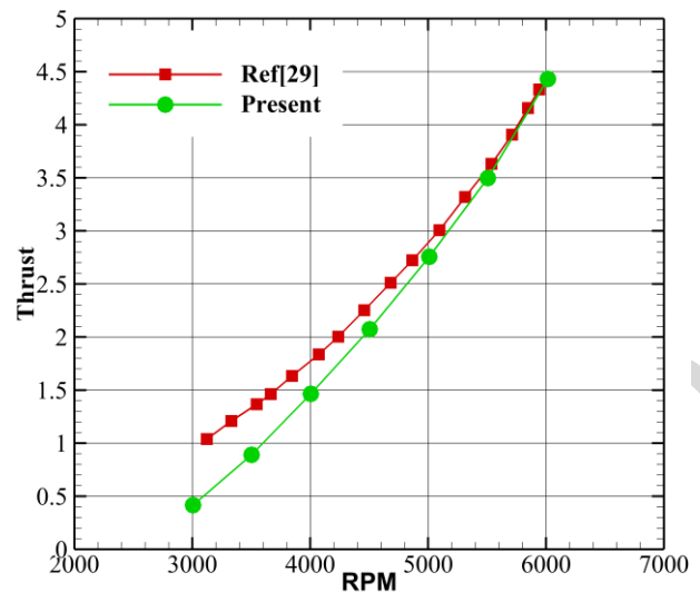
شکل ۱۶- اعتبارسنجی شبیه‌سازی با مرجع [۲۹].
