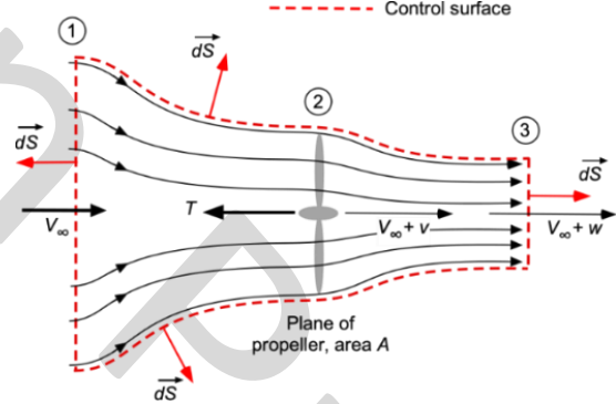
شکل ۱۲- طرحواره عبور جریان سیال از اطراف ملخ
