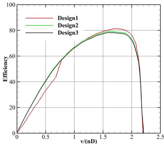
شکل ۷- مقایسه بازدهی ملخ‌ها بر حسب طول بی بعد شده ملخ.
