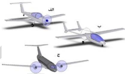
شکل ۴- چیدمان‌های: الف)پیش‌کشنده ب)هل‌دهنده ج) چندموتوره [۶].
