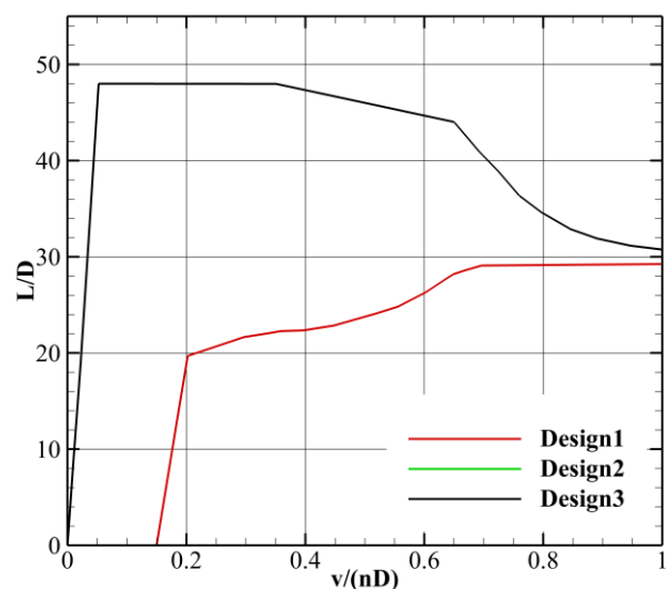
شکل ۱۰- مقایسه نیرو برا به پسا ملخها بر حسب طول بی بعد شده ملخ.
