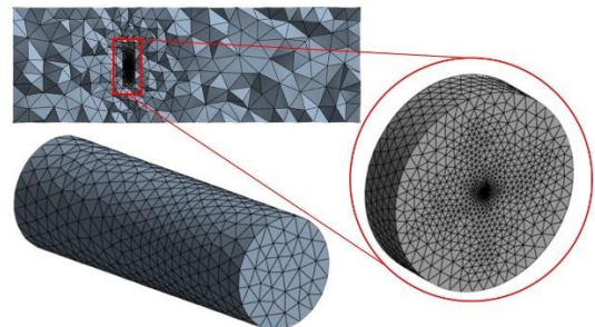
شکل ۱۳- شبکه بندی انجام شده.
