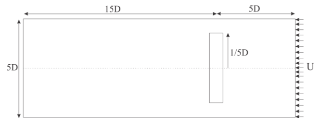
شکل ۱۳- دامنه حل.
