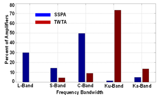
شکل ۴- توزیع TWTAها و SSPAها براساس فرکانس
