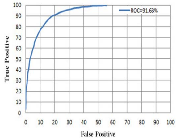
شکل ۸- نمودار ROC.
