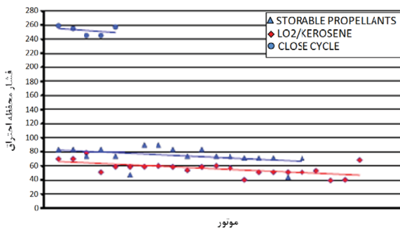
شکل (۳): محدوده فشار محفظه موتورها به تفکیک پیشران.
